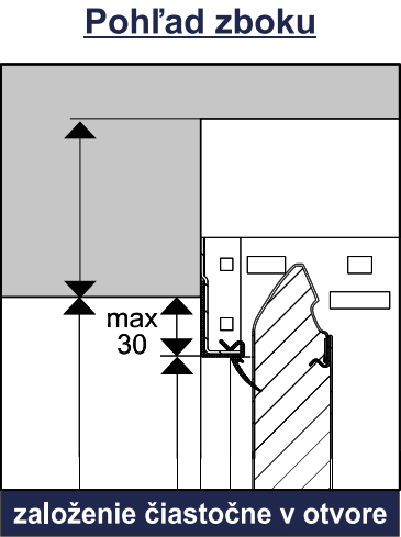
Založenie prekladového profilu
