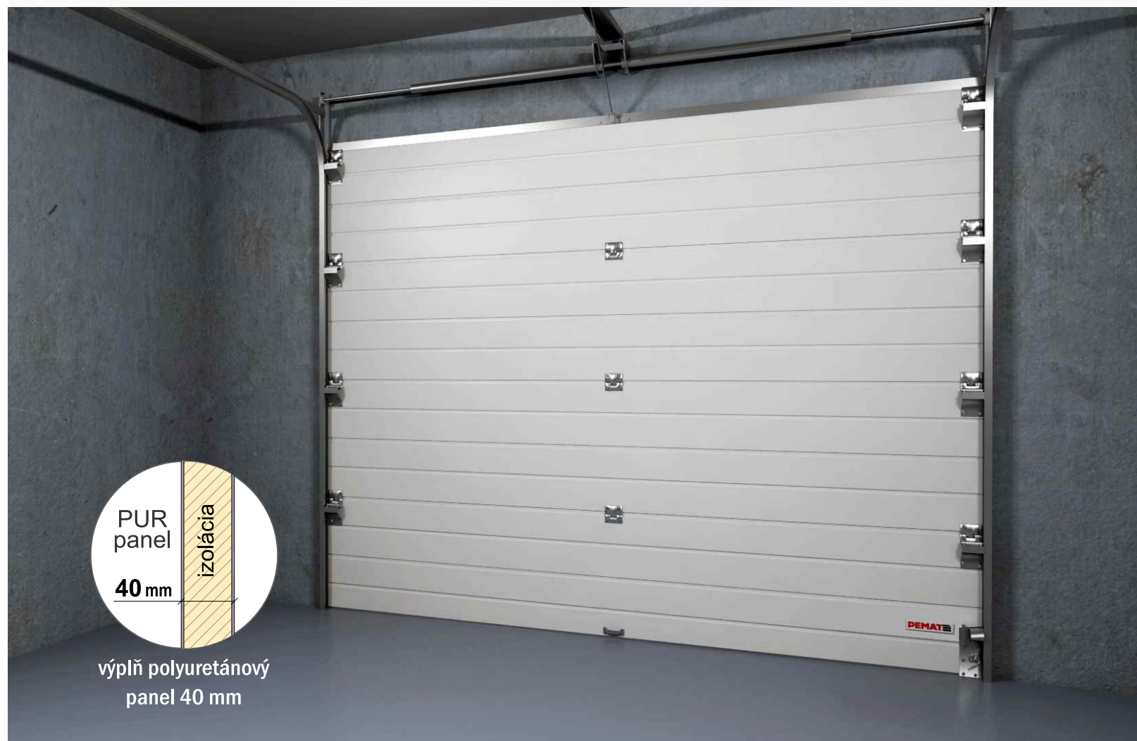
Vnútorný pohľad na sekčnú garážovú bránu so šírkou 2,5 m
