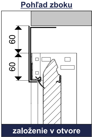
Založenie prekladového profilu
