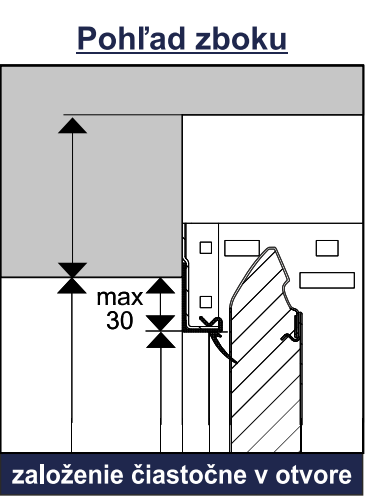
Založenie prekladového profilu
